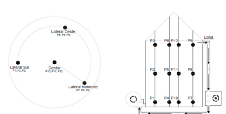
Figura 1. Sistema de medição da concentração de fosfina instalado no silo com mangueiras de medições ao longo dos cabos de termometria na lateral Sul, lateral Oeste, lateral Nordeste e centro do silo. Cambé, PR, 2020.
